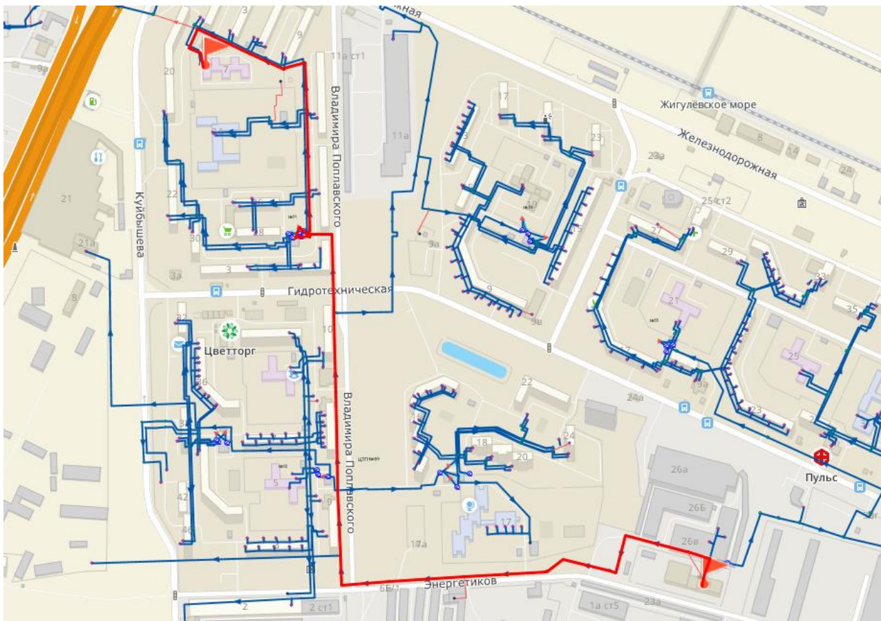
Рисунок 2.31 - Путь теплоносителя по направлению от котельной № 8 до потребителя «ул. Железнодорожная
