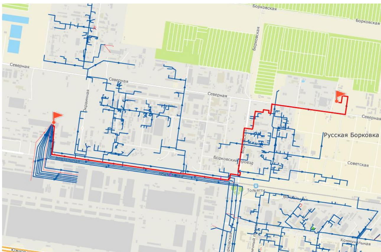
Рисунок 2.5 - Путь теплоносителя по направлению от ТЭЦ ВАЗ до потребителя «ул. Северная 10»
