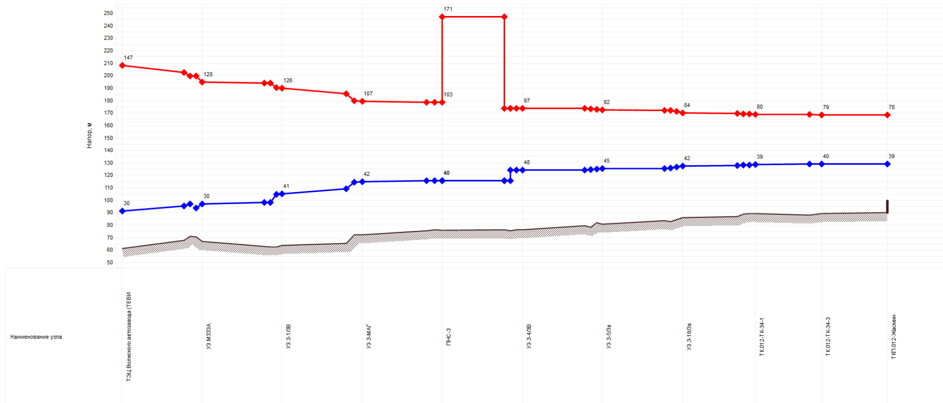
Рисунок 2.12 - Пьезометрический график от ТЭЦ ВАЗ до потребителя «ул. Автостроителей 84а»
