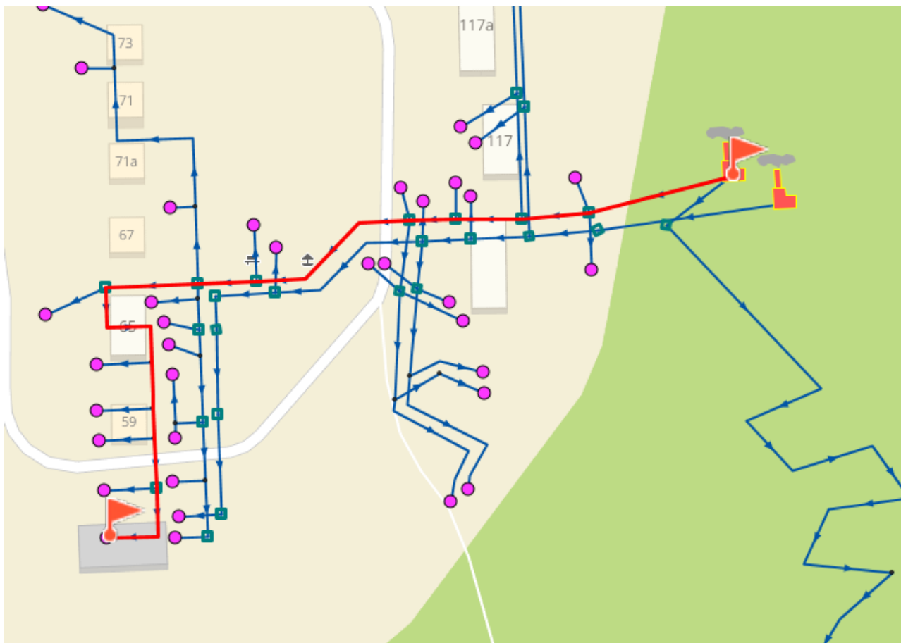
Рисунок 2.27 - Путь теплоносителя по направлению от Котельной №3 до потребителя «ул.Санаторная 55»
