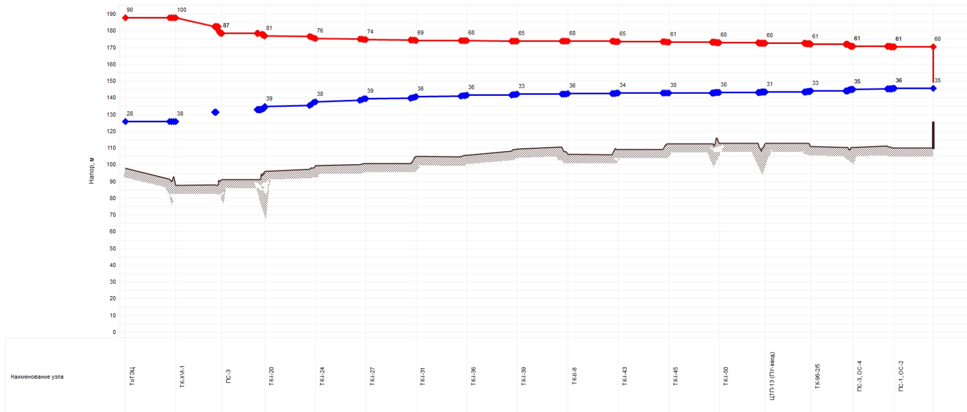
Рисунок 2.20 - Пьезометрический график от Тольяттинской ТЭЦ до потребителя «ул. Ушакова 62»
