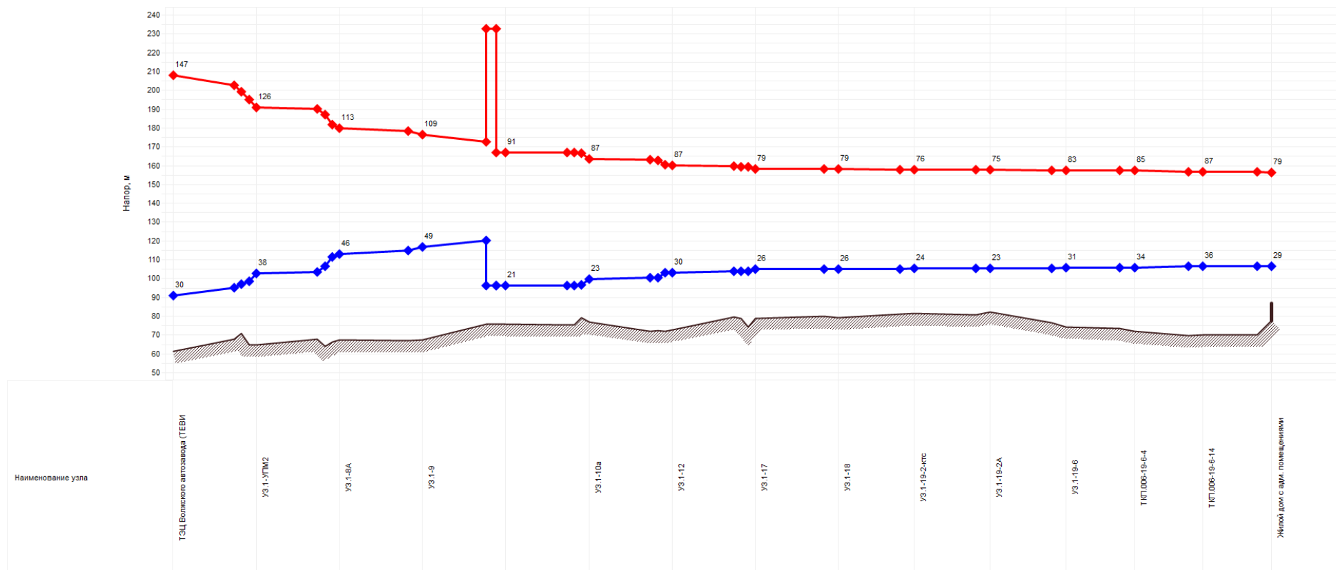
Рисунок 2.8 - Пьезометрический график от ТЭЦ ВАЗ до потребителя «Московский пр., 59»
