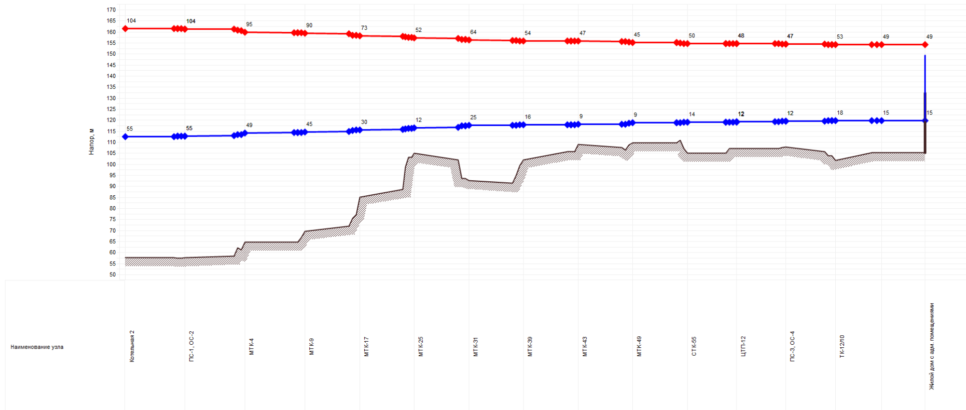
Рисунок 2.22 - Пьезометрический график от Котельной №2 до потребителя «ул.Коммунистическая 13»
