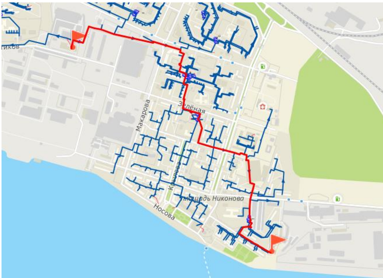
Рисунок 2.33 - Путь теплоносителя по направлению от котельной № 8 до потребителя «ул. Никонова 38»
