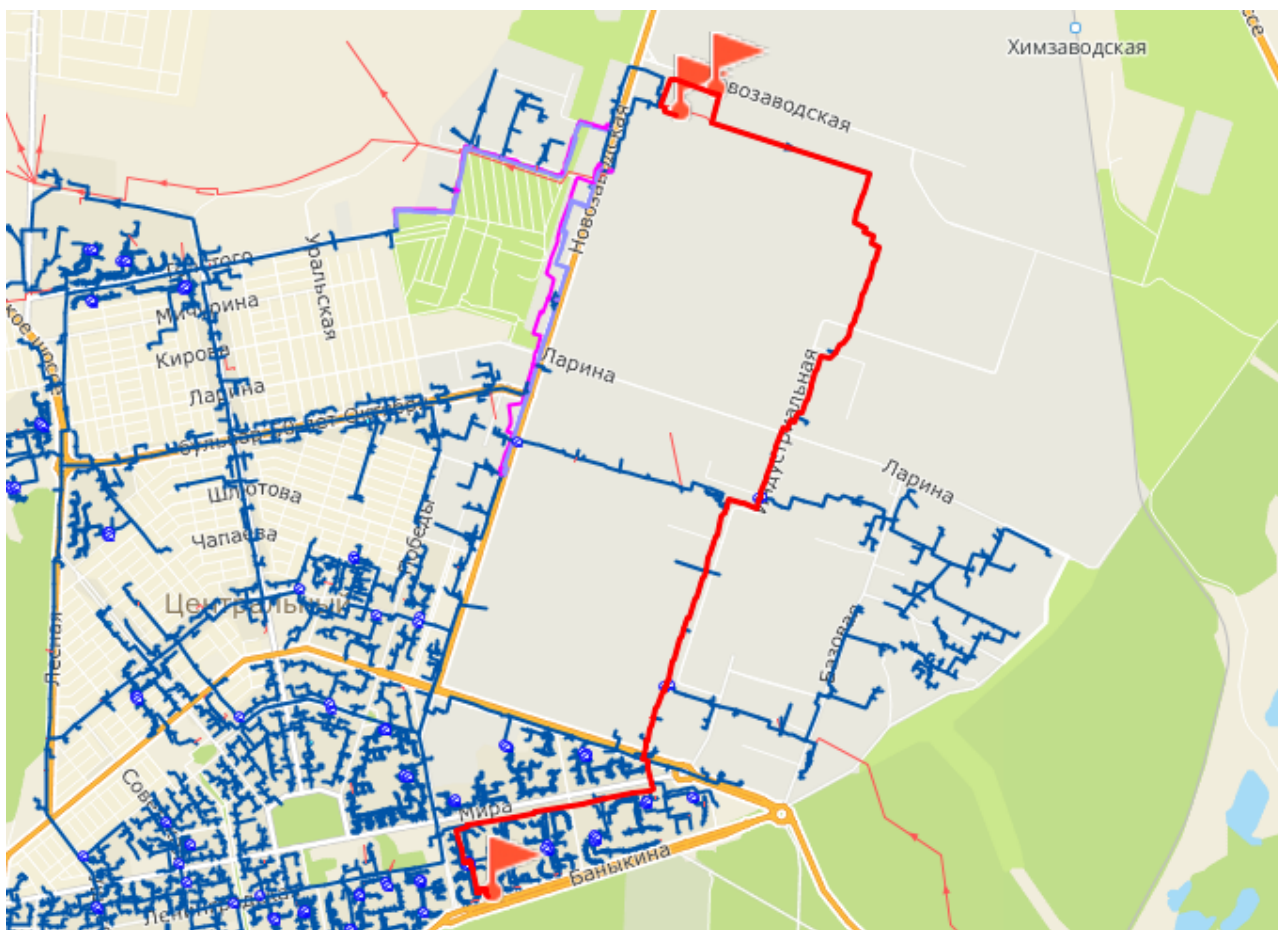
Рисунок 2.15 - Путь теплоносителя по направлению от Тольяттинской ТЭЦ до потребителя «ул. Баныкина, 38»
