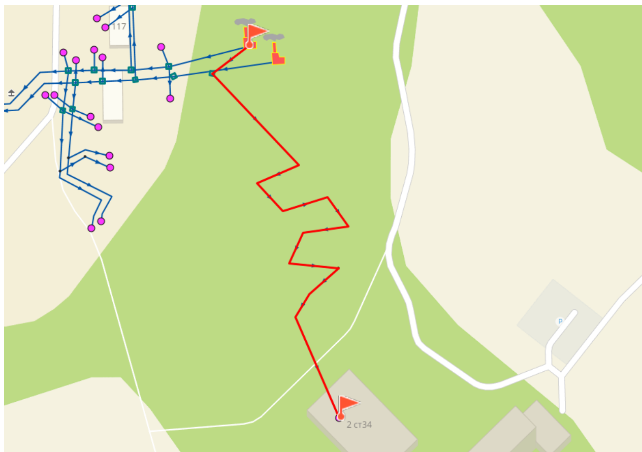
Рисунок 2.25 - Путь теплоносителя по направлению от Котельной №3 до потребителя «Лесопарковое шоссе 2»
