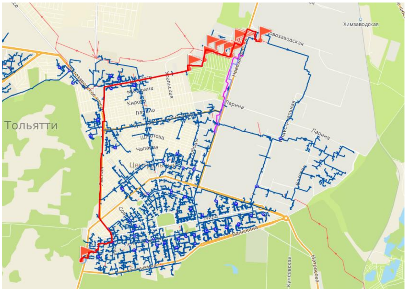
Рисунок 2.17 - Путь теплоносителя по направлению от Тольяттинской ТЭЦ до потребителя «ул. Родины 1д»
