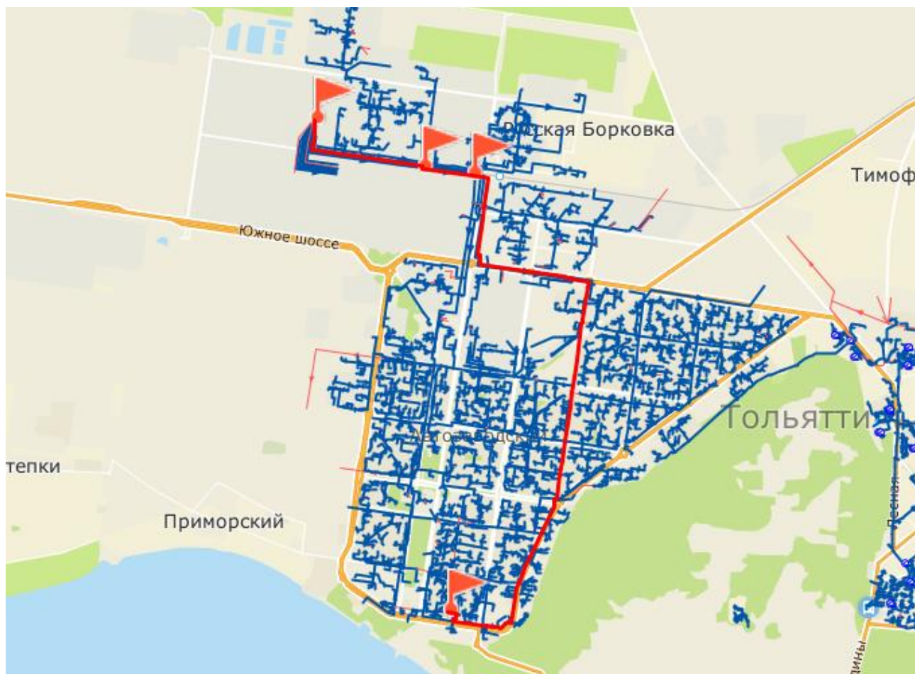
Рисунок 2.9 - Путь теплоносителя по направлению от ТЭЦ ВАЗ до потребителя «ул. Спортивная 10»
