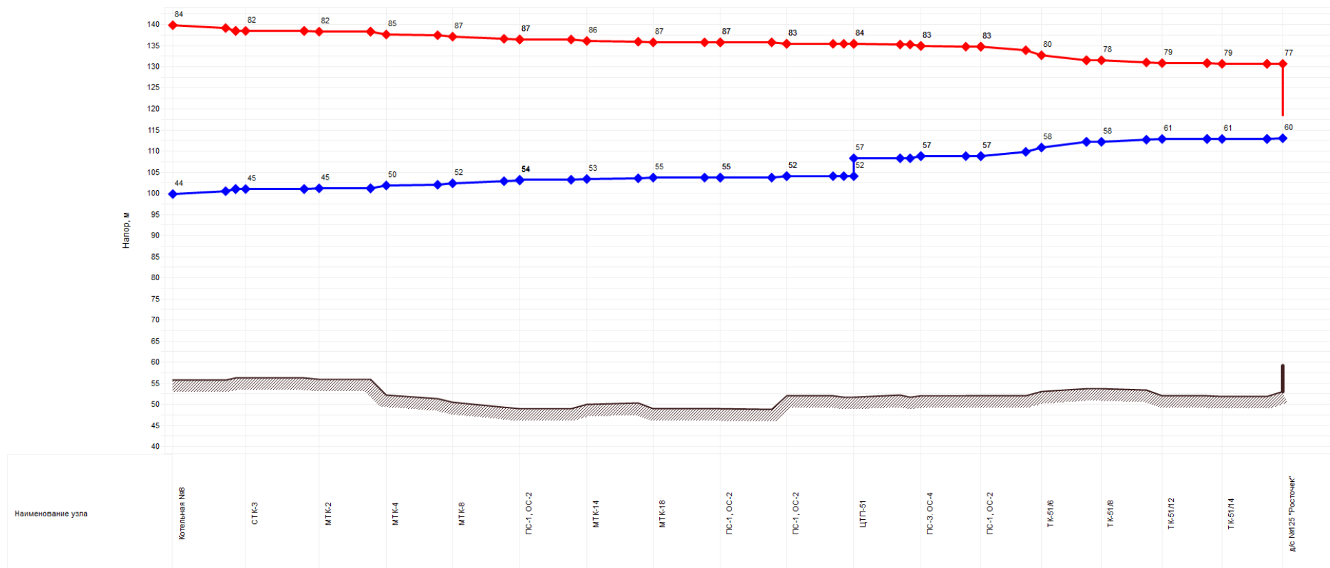
Рисунок 2.32 - Пьезометрический график от котельной № 8 до потребителя «ул. Железнодорожная 7»
