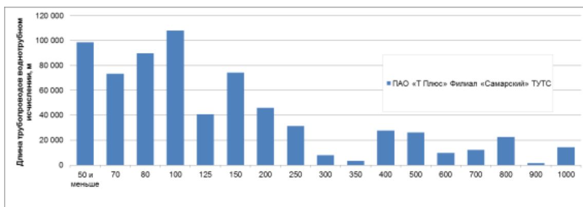
Рисунок 1.6 - Распределение протяженности трубопроводов тепловых сетей ТУТС ПАО «Т Плюс» по диаметру
