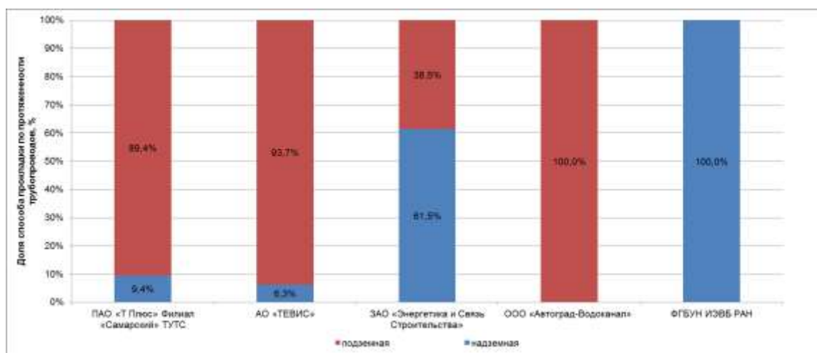
Рисунок 1.5 - Распределение долей способа прокладки по протяженности трубопроводов, %
