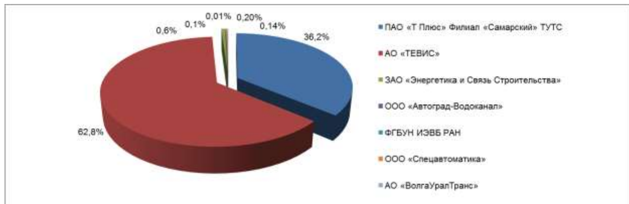
Рисунок 1.3 - Распределение материальной характеристики тепловых сетей по теплоснабжающим организациям г.о. Тольятти
