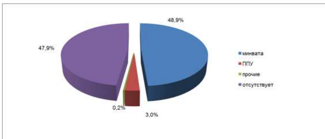
Рисунок 1.8 - Распределение суммарной протяженности тепловых сетей по виду тепловой изоляции
