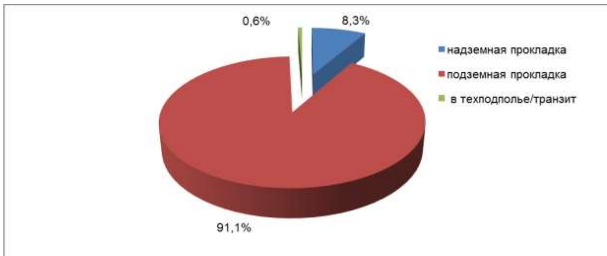
Рисунок 1.4 - Распределение суммарной протяженности тепловых сетей по способам прокладки
